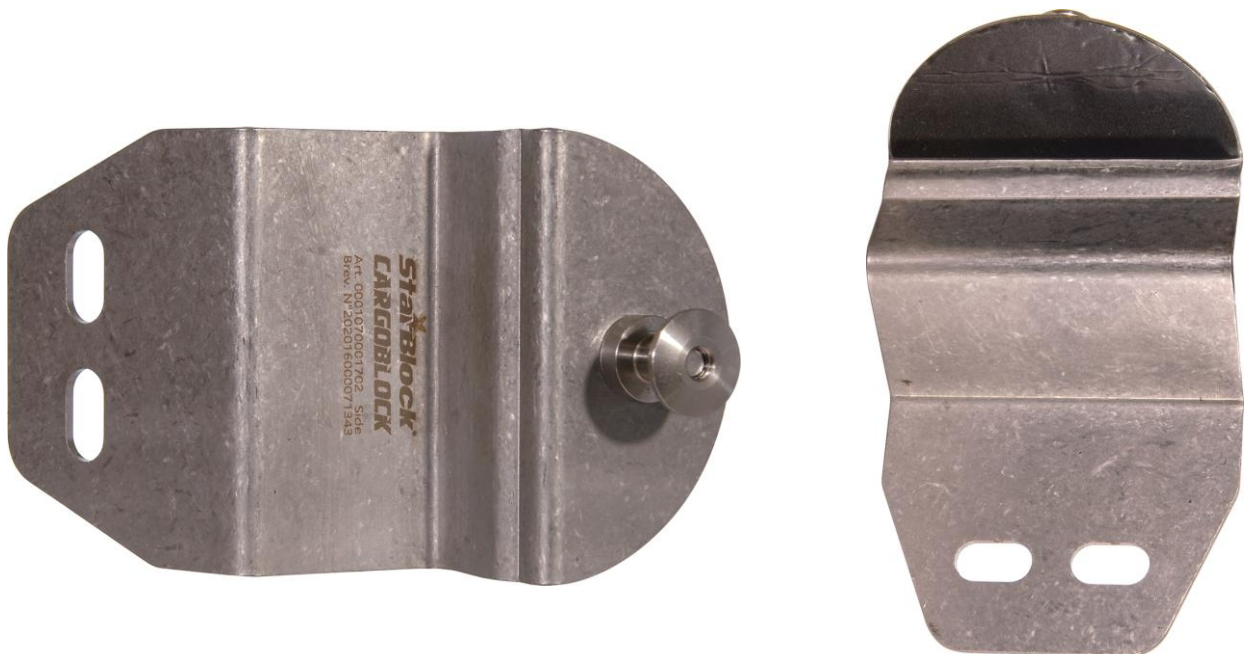
4- Plaque de fixation de la porte latérale
